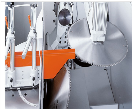
Uithoekzaagmachine AKS 134/00
