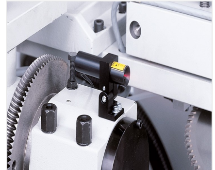
Uithoekzaagmachine AKS 134/00
