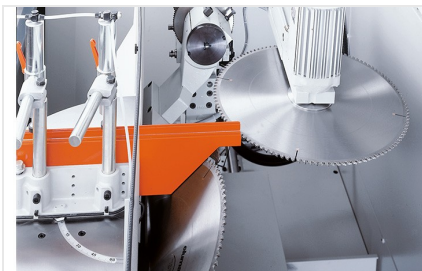
Uithoekzaagmachine AKS 134/00
