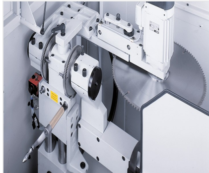
Uithoekzaagmachine AKS 134/00
