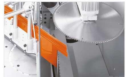
Uithoekzaagmachine AKS 134/00
