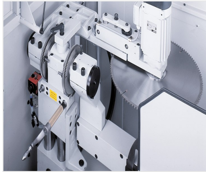
Uithoekzaagmachine AKS 134/00
