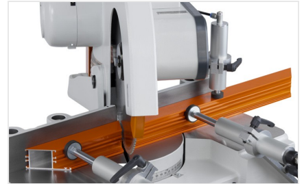
Troncatrice per tagli obliqui MGS 73/33
