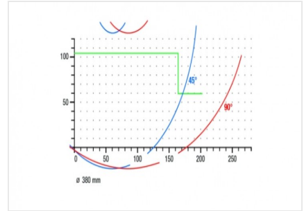
Troncatrice per tagli obliqui MGS 73/33
