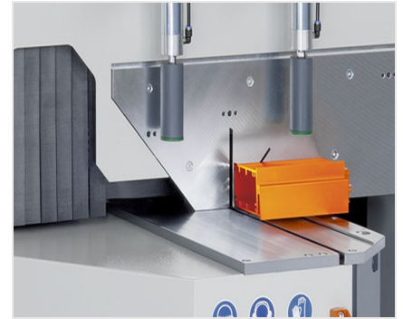
Troncatrice per tagli obliqui MGS 105
