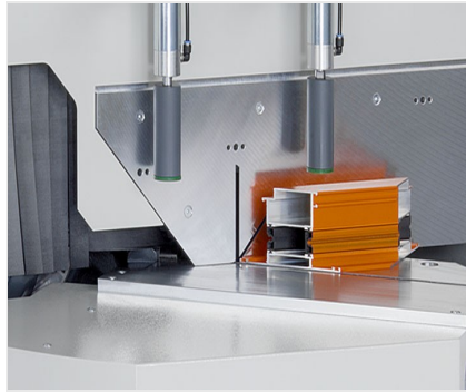
Troncatrice per tagli obliqui MGS 105
