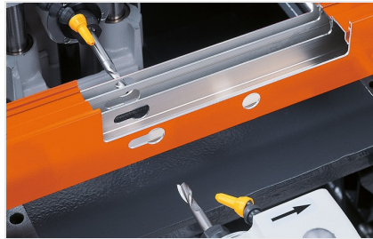
Pantografo a 2 mandrini KF 78/23
