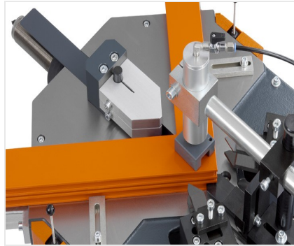
Cianfrinatrice per angoli EP 120
