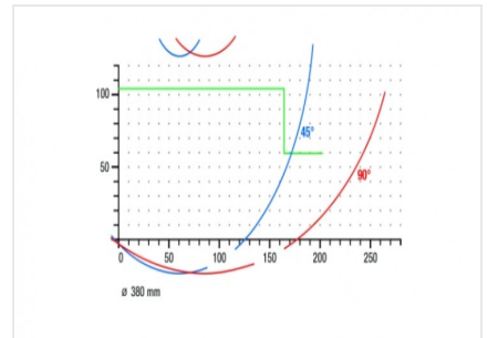
Troncatrice bilama DG 79 Diagramma di taglio DG 79
