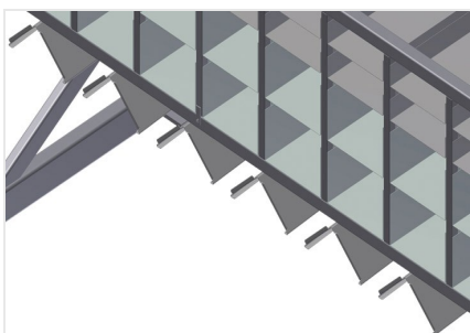
Supporto angolare
