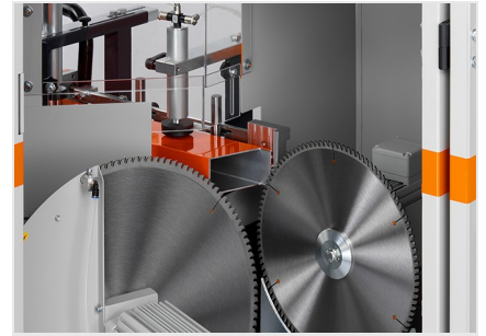
Troncatrice intestatrice AKS V-550
