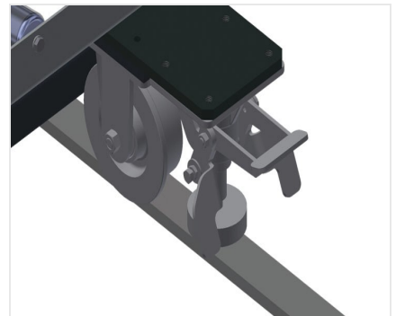
行走单元 带凸缘滚轮和驻车制动器的行走装置
