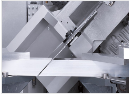
型材加工中心 SBZ 630
