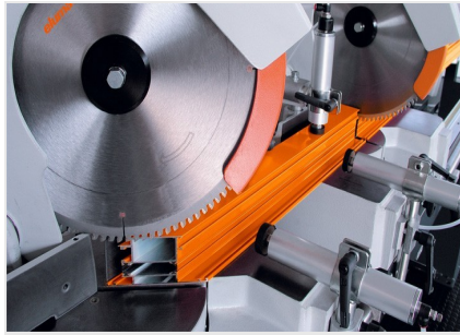
双头斜榫切割机DG 79
