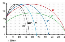
双头斜榫切割机DG 244
