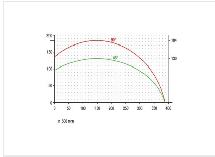
双头斜榫切割机DG 142
