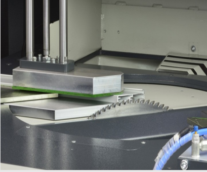
Kesme Merkezi SBZ 616/02
