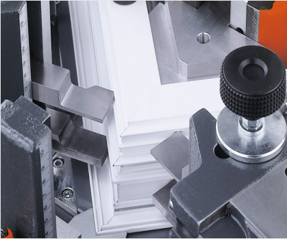
Köşe bağlantı presi EP 124
