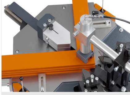
Köşe bağlantı presi EP 120
