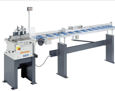
Настольная пила TS 161/21 + MMS 200
