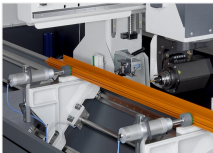
Обрабатывающий центр SBZ 122/74
