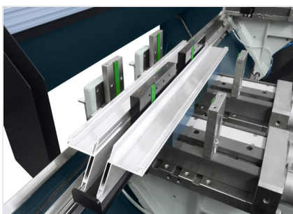
Обработывающий центр SBZ 122/74
