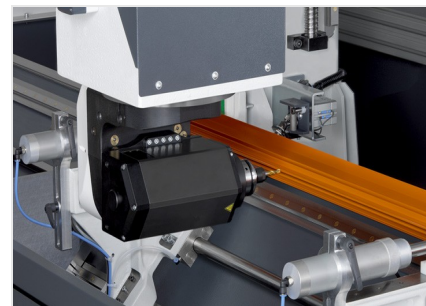
Регулировка угла с помощью оси A
