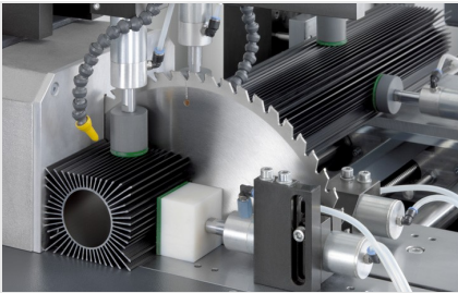
Пильный автомат SAS 142/43
