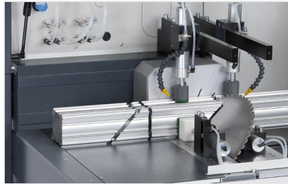
Пильный автомат SAS 142/43
