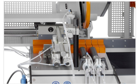
Пильный автомат SA 73/36
