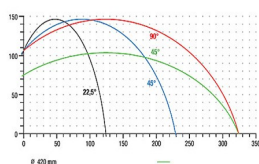
Ускоренная пила MGS 105
