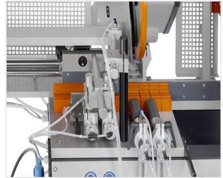
Máquina de corte automática SA 73/36
