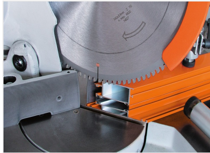
Máquina de corte angular MGS 73/33
