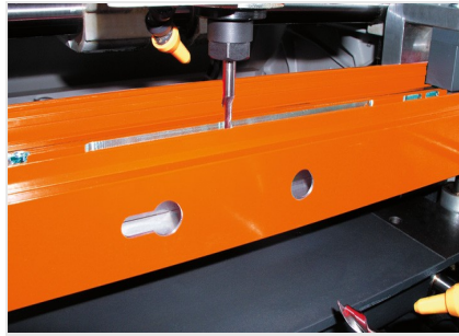
Fresa-copiadora de 2 cabeças KF 78/23
