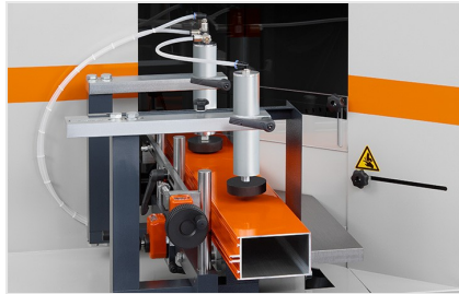
Máquina de corte e malhete AKS V-550
