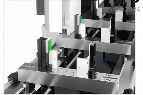
Centrum obróbcze profili SBZ 141
