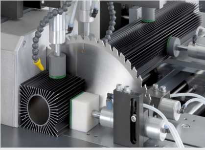
Automat do cięcia SAS 142/43
