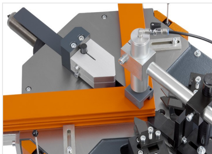
Zaciskarka do naroży EP 120
