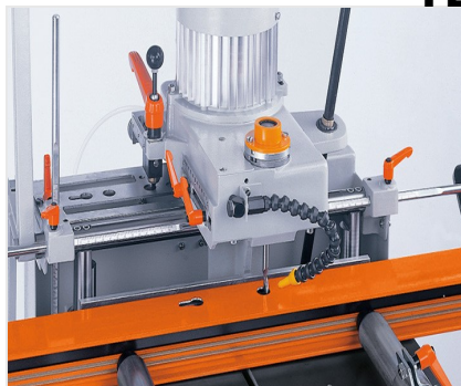
Jednowrzecionowa frezarko-kopiarka AS 70/44
