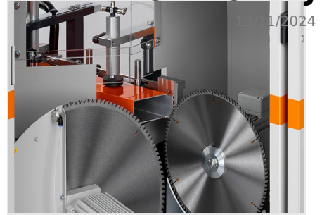
Piły do wycięć klinowych AKS V-550
