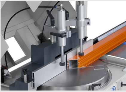
Tafelzaag TS 161/30
