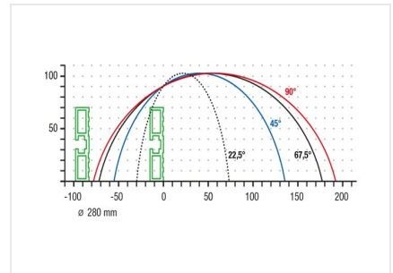
Tafelzaag TS 161
