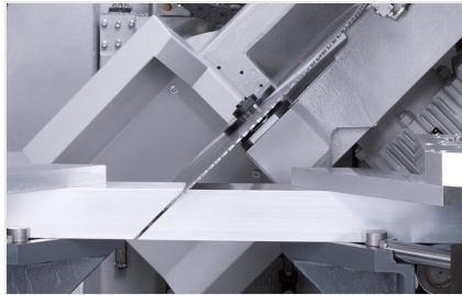
Profielbewerkingscentrum SBZ 631
