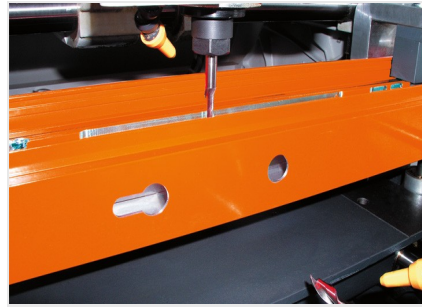
Tweespindel- kopieerfreemACHINE KF 78/23
