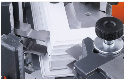
Hoekverbindingspers EP 124
