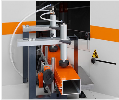
Uithoekzaagmachine AKS V-550
