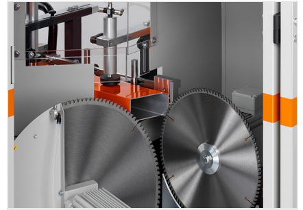
Uithoekzaagmachine AKS V-550
