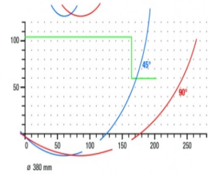
Troncatrice per tagli obliqui MGS 73/33
