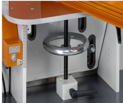
Fresatrice intestatrice AF 223/01
