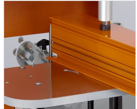
Fresatrice intestatrice AF 223/01
