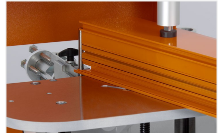
Fresatrice intestatrice AF 223/01
