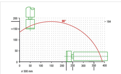
Scie automatique 142/42
