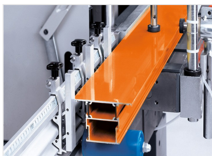
Fraiseuse à copier mono- broche AS 170/10
