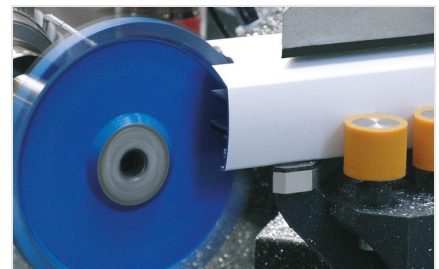
Centro de mecanizado de barras SBZ 631
