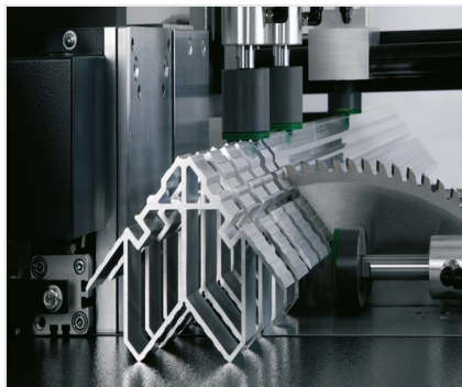
Tronzadora automática SA 142/38
