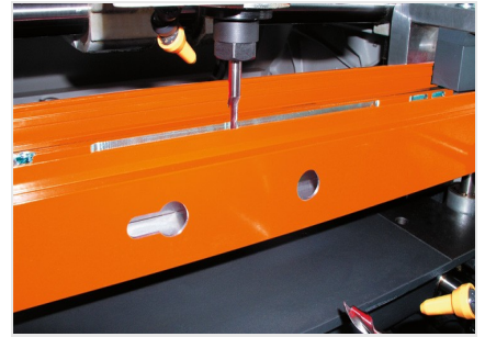
Copiadora fresadora doble KF 78/23
