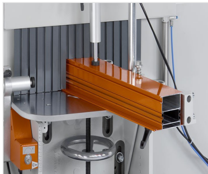
Fresadora retestadora AF 223/01
