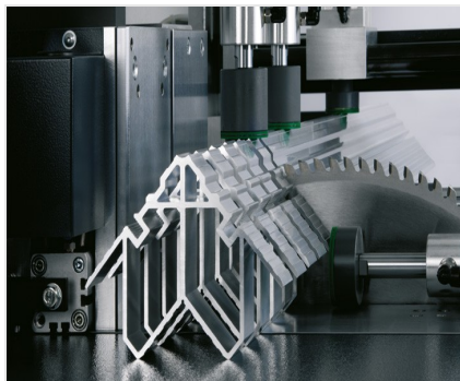
Automatic saw SA 142/38
