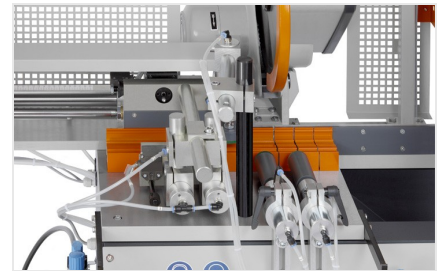
Sägeautomat SA 73/36
