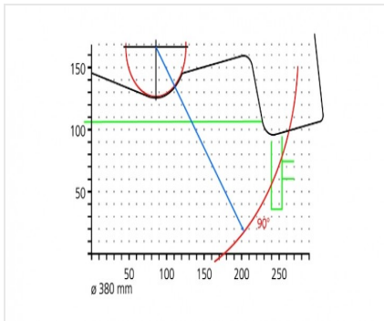
Sägeautomat SA 73/36
