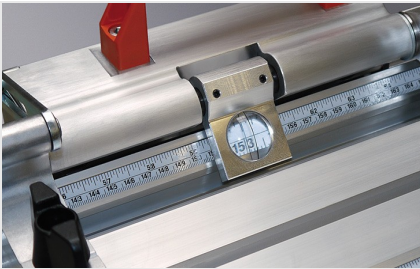
Anschlag- und Mess- System MMS 100
