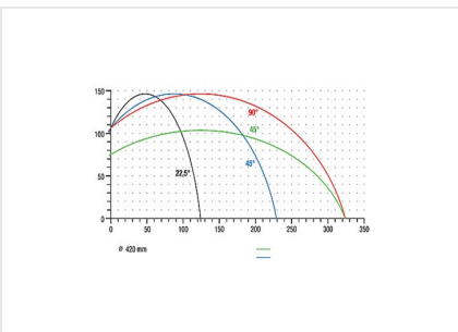
Gehrungssäge MGS 105
