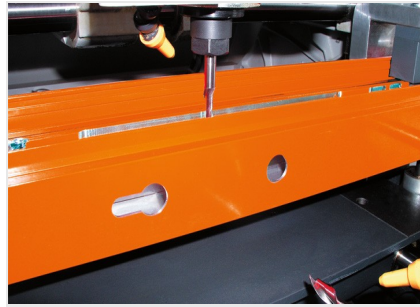
2-Spindel-Kopierfräse KF 78/23
